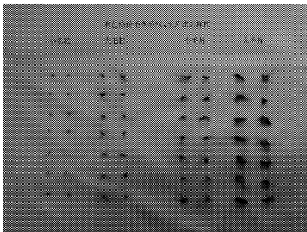
图 A.1 有色涤纶毛条毛粒、毛片比对样照
